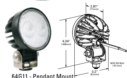
64G11 - Pendant Mount
